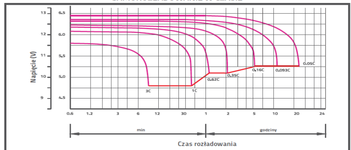
CHARAKTERYSTYKA ROZŁADOWANIA
